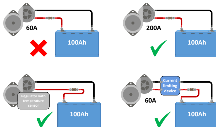
Laddning med växelströmsgenerator
